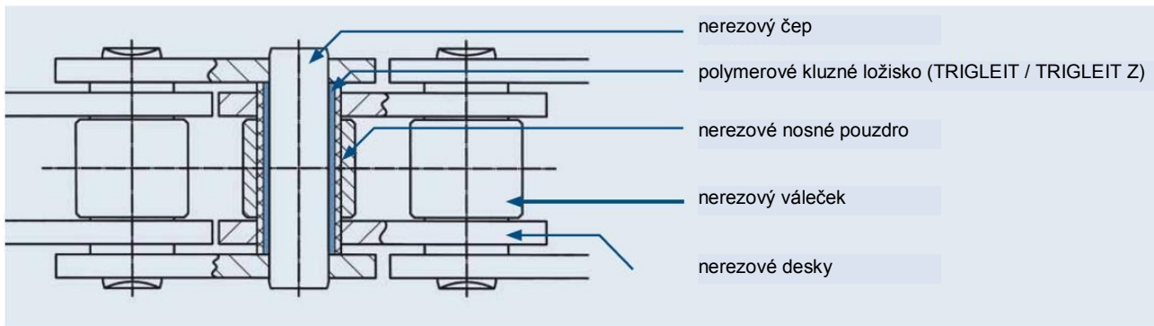
Vysoce zatížitelná polymerová kluzná ložiska TRIGLEIT
